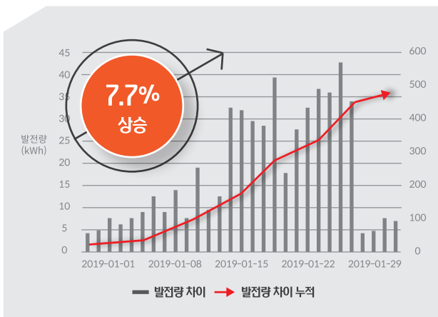
동서발전 당진화력 (주)에코센스 SunRobot 효율 시험 결과
