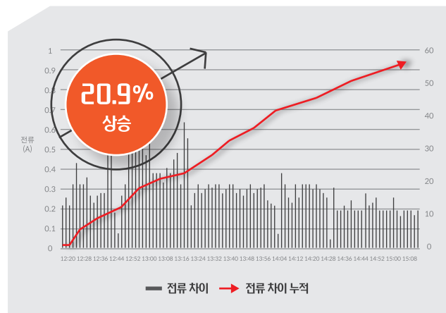
한화큐셀 영암산업 (주)에코센스 SunRobot 효율 시험 결과
